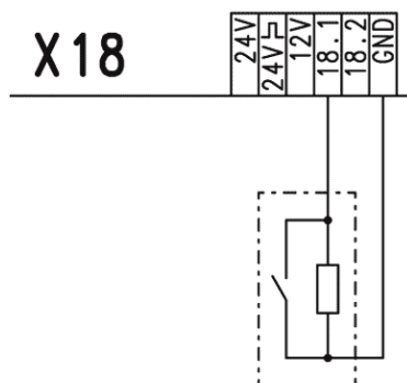
Schaltleiste 8K2 als Einzugssicherung einfach
