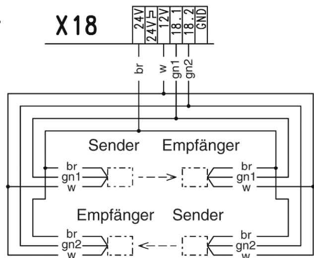
Raytector Lichtschranke oder Optische Schaltleiste als Einzugssicherung zweifach
