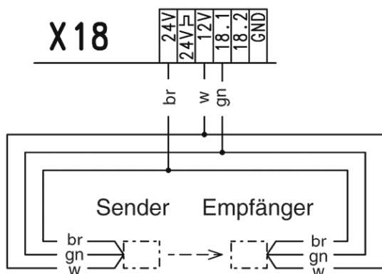
Raytector Lichtschranke oder Optische Schaltleiste als Einzugssicherung einfach
